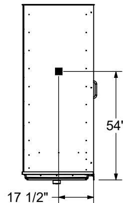
LEFT SIDE VIEW / VUE DE CÔTÉ GAUCHE
