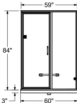
FRONT VIEW / VUE DE FACE
