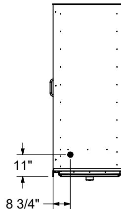
LEFT SIDE VIEW / VUE DE CÔTÉ GAUCHE
